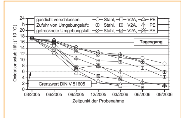
Abb. 53: Oxidationsstabilität (DIN EN 14112) von Rapsölkraftstoffproben aus High-Oleic-Sommerraps unter dem Einfluss unterschiedlicher Lagerungsbedingungen bei ungeschützter Lagerung im Freien
