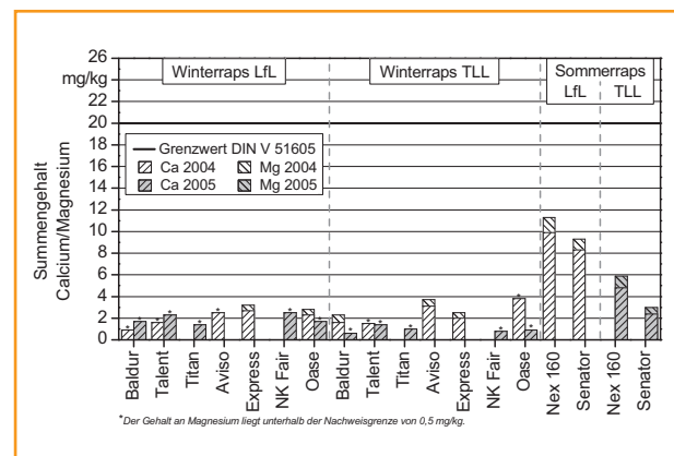
Abb. 28: Summengehalt an Calcium und Magnesium (DIN EN 14538) der Ölproben verschiedener Rapssorten von unterschiedlichen Standorten der Erntejahre 2004 und 2005
