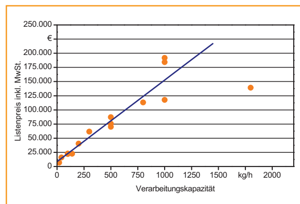
Abb. 71: Listenpreise von Seihstabs-Schneckenpressen in Abhängigkeit von der Verarbeitungskapazität (inkl. MwSt.)
