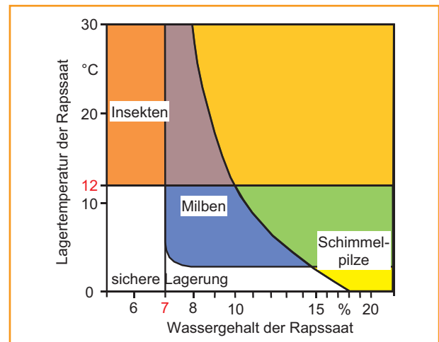
Abb. 39: Befall eines Rapslagers mit Insekten, Milben und Schimmelpilzen in Abhängigkeit des Wassergehalts und der Lagertemperatur der Rapssaat (verändert nach JACOBSEN, E. E. (1995) [41])
