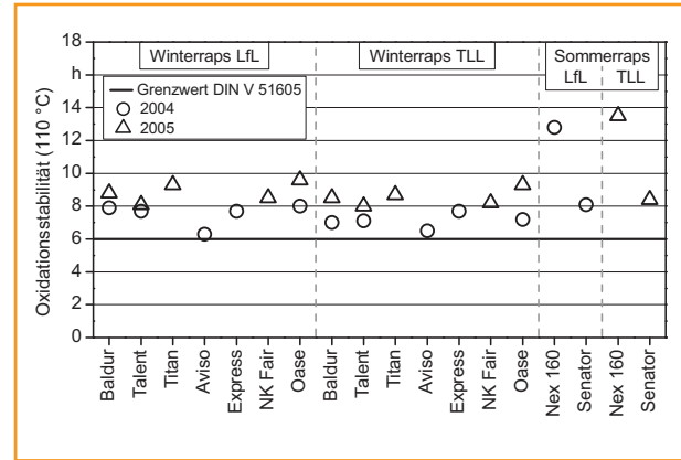
Abb. 27: Oxidationsstabilität (DIN EN 14112) der Ölproben verschiedener Rapssorten von unterschiedlichen Standorten der Erntejahre 2004 und 2005
