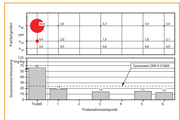
Abb. 49: Gesamtverschmutzung und Partikelgrößenverteilung in Rapsöl vor und nach Filtration mit einem Beutelfilter 2-AXL-1 µm des Herstellers Filtrertechnik Jäger
