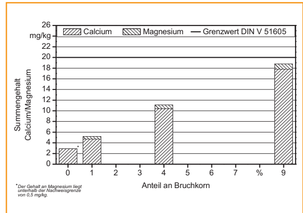
Abb. 37: Summengehalt an Calcium und Magnesium (DIN EN 14538) der Ölproben aus Rapssaat mit verschiedenen Anteilen an Bruchkorn (verändert nach DIETL, G. (2004) [24])
