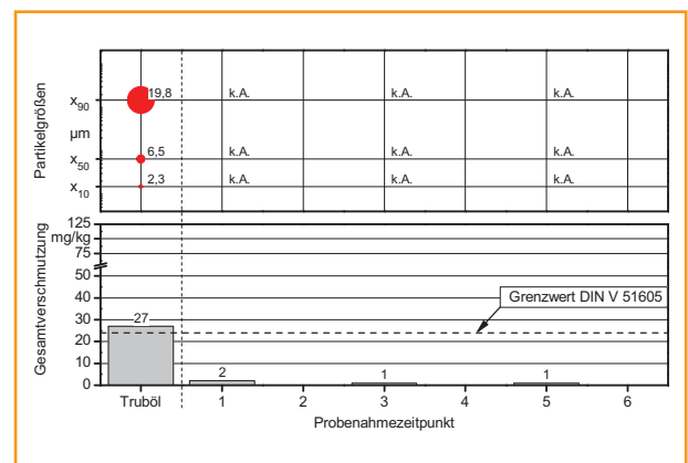
Abb. 45: Gesamtverschmutzung und Partikelgrößenverteilung in Rapsöl vor und nach Filtration mit einem SUPRADisc SD K300 des Herstellers Pall SeitzSchenk
