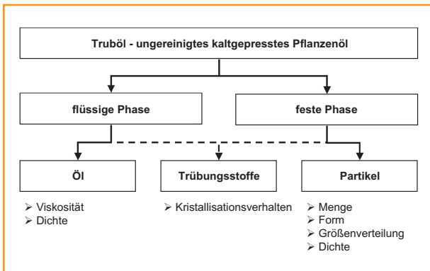
Abb. 11: Charakterisierung von Trüböl
