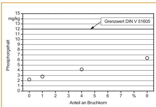
Abb. 36: Phosphorgehalt (DIN EN 14107) der Ölproben aus Rapssaat mit verschiedenen Anteilen an Bruchkorn (verändert nach DIETL, G. (2004) [24])
