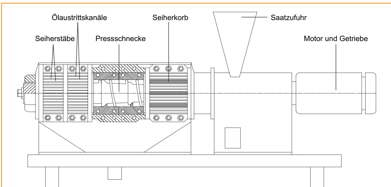
Abb. 8: Seiherstab-Schneckenpresse
