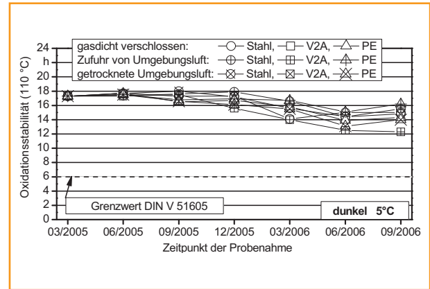
Abb. 54: Oxidationsstabilität (DIN EN 14112) von Rapsölkraftstoffproben aus High-Oleic-Sommerraps unter dem Einfluss unterschiedlicher Lagerungsbedingungen bei lichtgeschützter Lagerung und einer Temperatur von 5 °C
