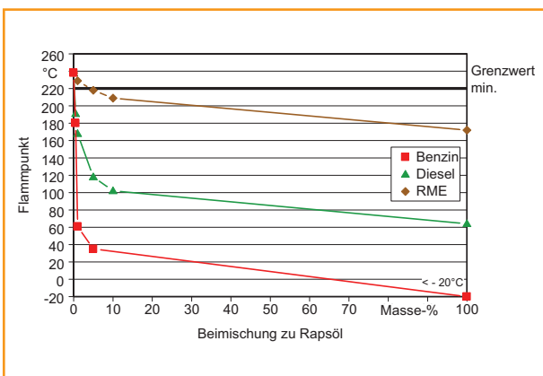
Abb. 55: Flammpunkt (DIN EN 22719) von Mischungen von Rapsölkraftstoff mit Benzol, Dieseldieselkraftstoff und Rapsölmethylester [60]
