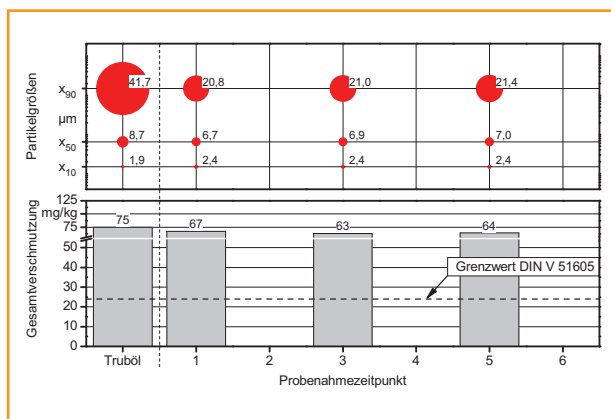
Abb. 47 Gesamtverschmutzung und Partikelgrößenverteilung in Rapsöl vor und nach Filtration mit einem Beutelfilter AP 1/1/1S-1S des Herstellers Amafilter
