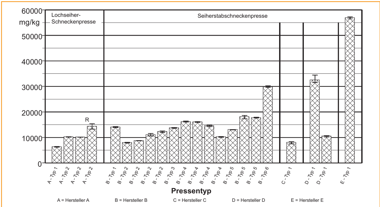
Abb. 13: Gesamtverschmutzung (in Anlehnung an DIN 51419-A) im ungereinigten Öl in Abhängigkeit vom Pressentyp [177]
