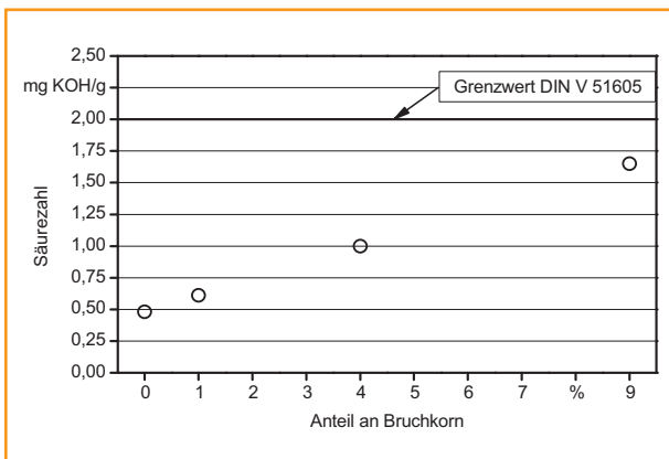
Abb. 35: Säurezahl (DIN EN ISO 660) der Ölproben aus Rapssaat mit verschiedenen Anteilen an Bruchkorn (verändert nach DIETL, G. (2004) [24])
