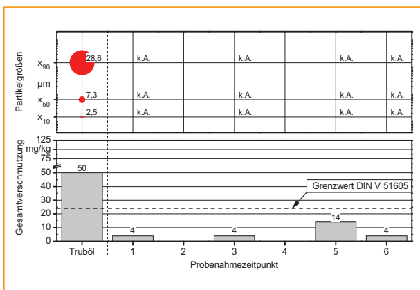
Abb. 43: Gesamtverschmutzung und Partikelgrößenverteilung in Rapsöl vor und nach Filtration mit einem Kerzenfilter EP 001-10-U-X4N des Herstellers Amafilter
