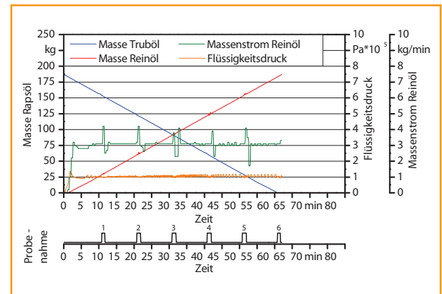
Abb. 48: Filtration von Rapsöl mit einem Beutelfilter 2-AXL-1 µm des Herstellers Filtrertechnik Jäger
