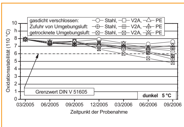
Abb. 52: Oxidationsstabilität (DIN EN 14112) von Rapsölkraftstoffproben aus Wintereraps unter dem Einfluss unterschiedlicher Lagerungsbedingungen bei lichtgeschützter Lagerung und einer Temperatur von 5 °C
