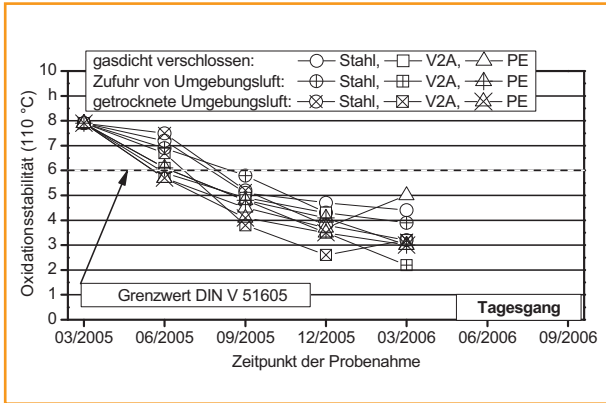
Abb. 50: Oxidationsstabilität (DIN EN 14112) von Rapsölkraftstoffproben aus Wintereraps unter dem Einfluss unterschiedlicher Lagerungsbedingungen bei ungeschützter Lagerung im Freien
