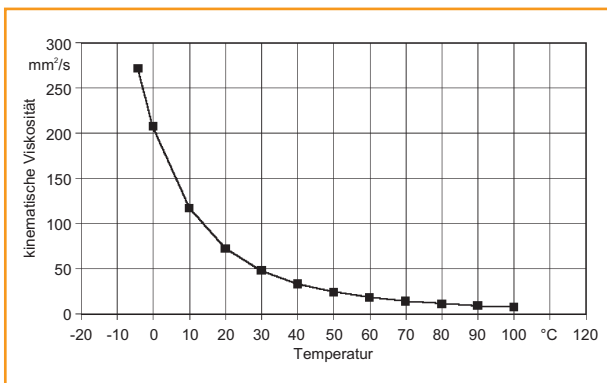
Abb. 12: Viskositäts-/Temperaturverhalten nach DIN 51562-1 (Ubbelohde) von kaltgepresstem Rapsöl [74]
