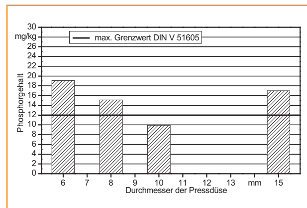
Abb. 41: Phosphorgehalt in Rapsöl in Abhängigkeit des Durchmessers der Pressdüse (nach WIDMANN, B. (1994) [76])
