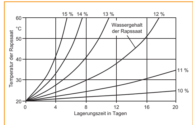
Abb. 38: Temperatur von Rapssaat (Selbsterhitzung) in Abhängigkeit von der Lagerdauer und dem Wassergehalt der Rapssaat (verändert nach JACOBSEN, E. E. (1995) [41])
