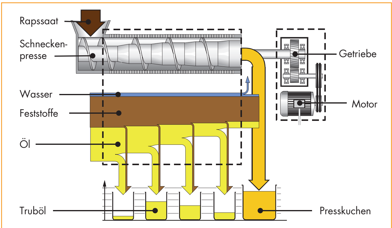
Abb. 10: Stoffflüsse bei der Ölpressung (verändert nach SCHEIN, C. (2003) [66])
