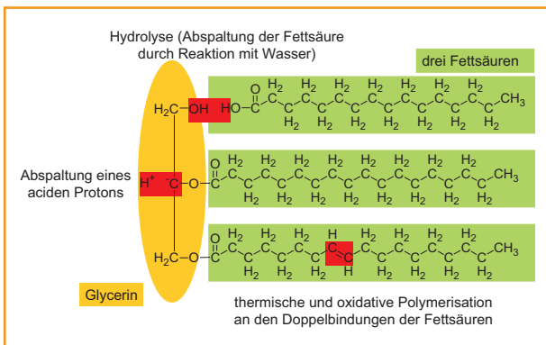
Abb. 60: Beispiele reaktiver Bindungen eines Triglycerids
