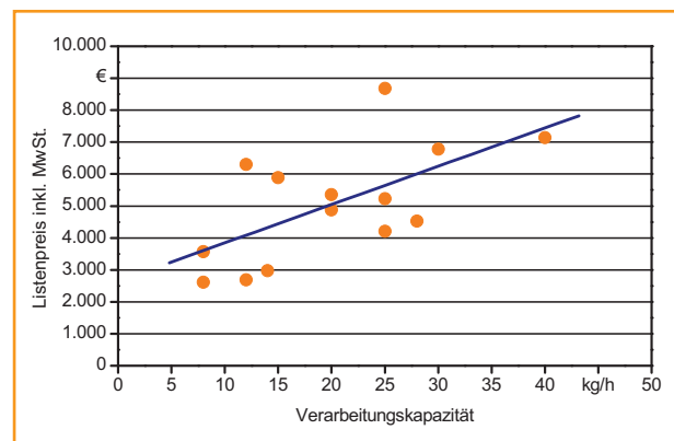
Abb. 70: Listenpreise von Lochseih-Schneckenpressen in Abhängigkeit von der Verarbeitungskapazität (inkl. MwSt.)
