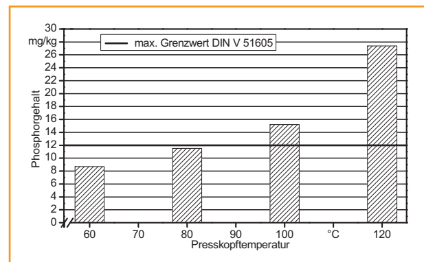
Abb. 40: Phosphorgehalt in Rapsöl in Abhängigkeit von der Presskopftemperatur (nach WIDMANN, B. (1994) [76])
