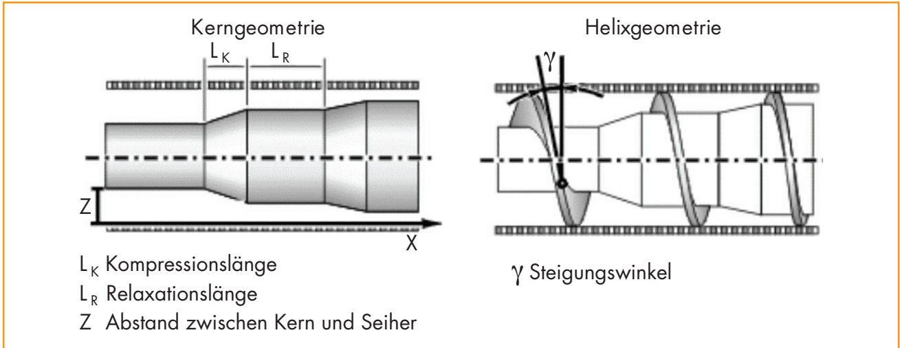
Abb. 9: Geometrie der Schneckenwelle einer Schneckenpresse – links: Geometrie des Kerns, rechts: Geometrie der Helix (nach SCHEIN, C. (2003) [66])
