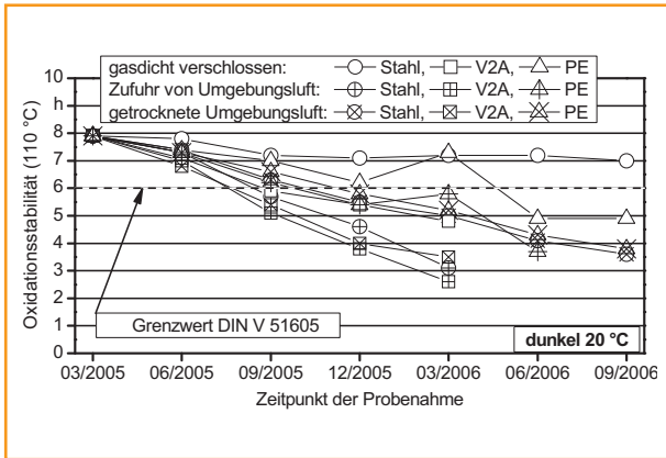
Abb. 51: Oxidationsstabilität (DIN EN 14112) von Rapsölkraftstoffproben aus Wintereraps unter dem Einfluss unterschiedlicher Lagerungsbedingungen bei lichtgeschützter Lagerung und einer Temperatur von 20 °C
