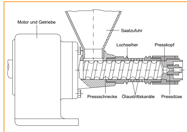
Abb. 7: Lochseiher-Schneckenpresse
